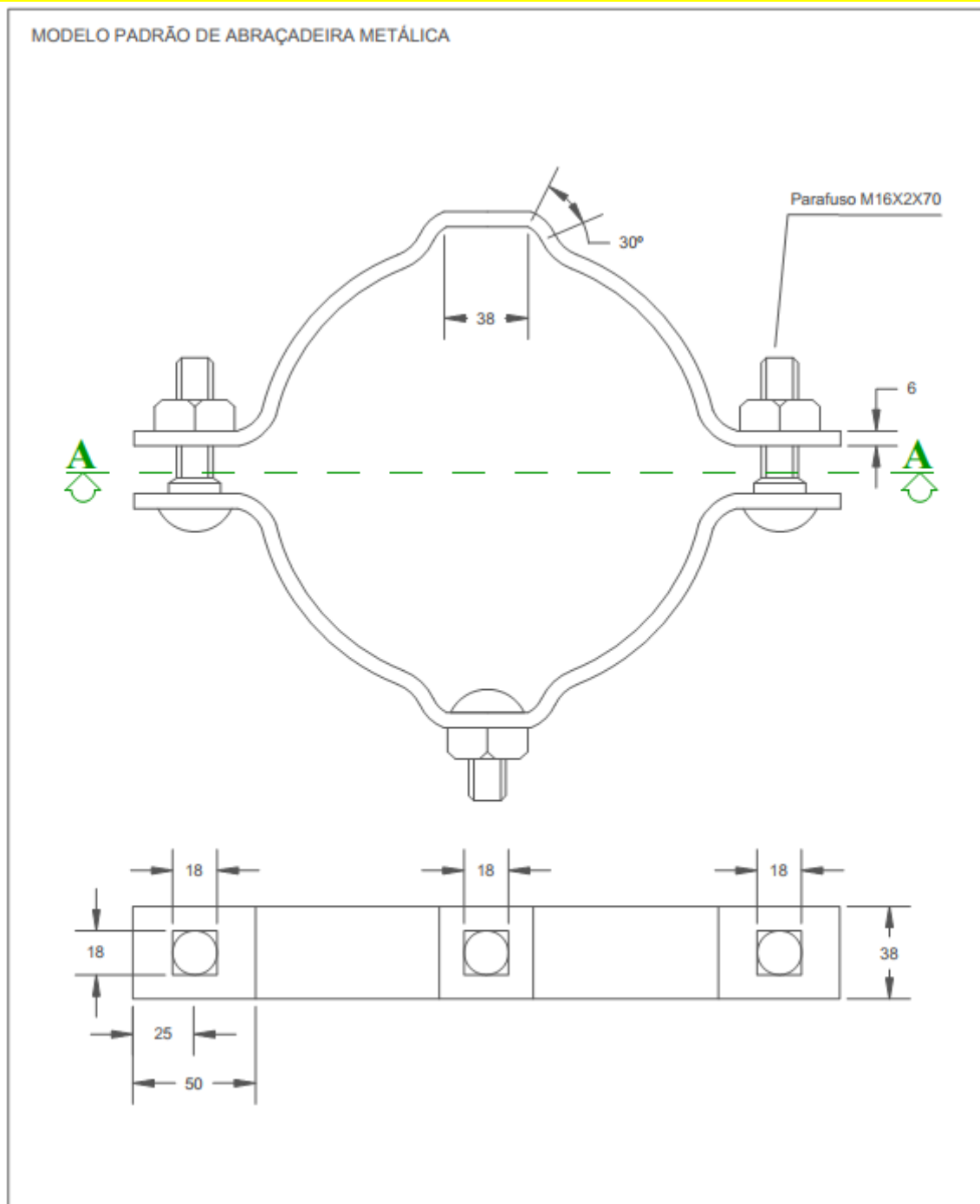
Figura 1 – Modelo das abraçadeiras de aço de 150 a 320mm.
